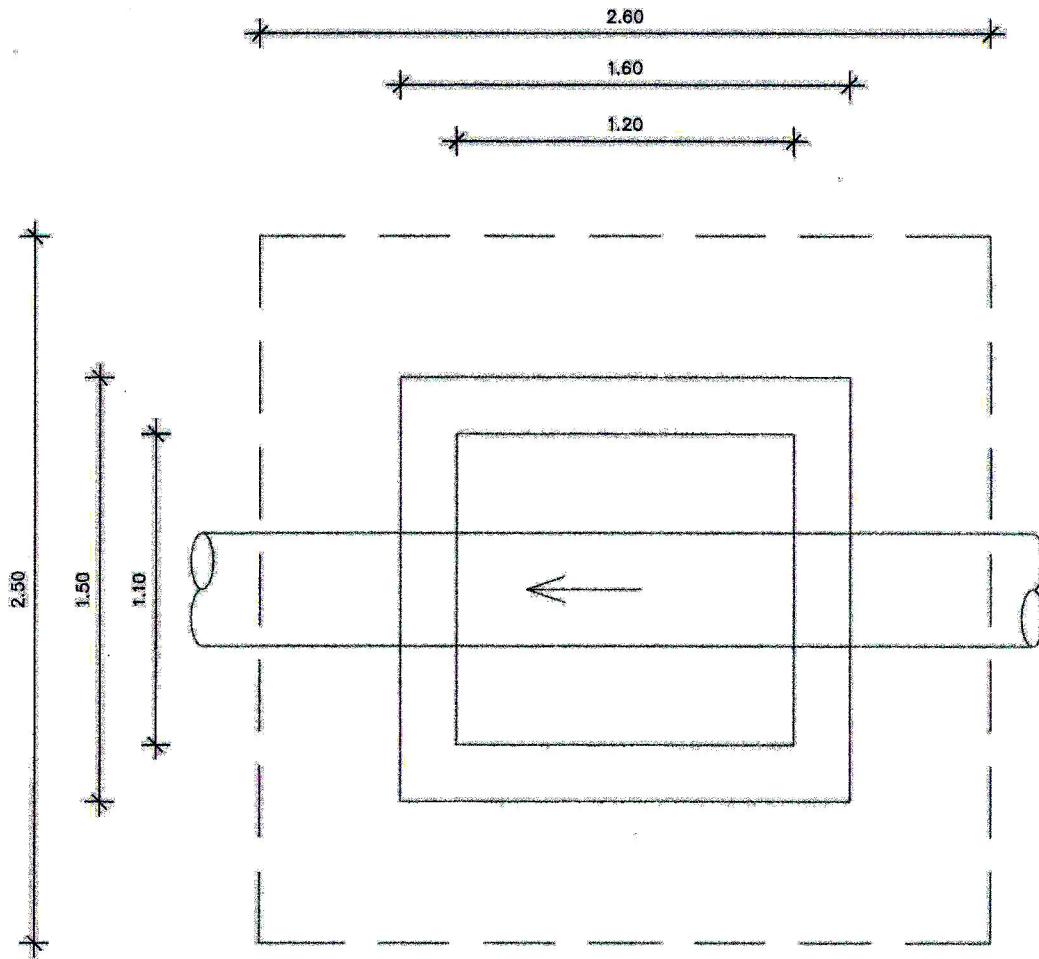
ΚΑΤΟΨΗ ΦΡΕΑΤΙΟΥ ΕΠΙΣΚΕΨΗΣ (ID>0.79)
