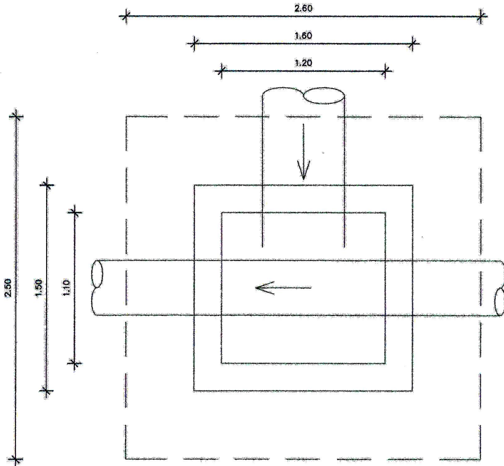
ΚΑΤΟΨΗ ΦΡΕΑΤΙΟΥ ΕΠΙΣΚΕΨΗΣ ΣΕ ΣΥΜΒΟΛΗ
