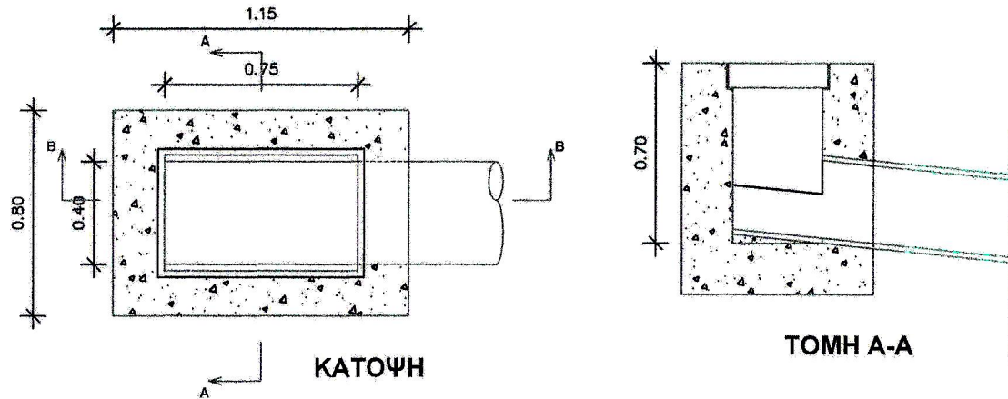
ΦΡΕΑΤΙΟ ΥΔΡΟΣΥΛΛΟΓΗΣ, ΤΟΠΟΘΕΤΟΥΜΕΝΟ ΚΑΘΕΤΑ ΣΤΟ ΟΡΙΟ ΤΗΣ ΟΔΟΥ
