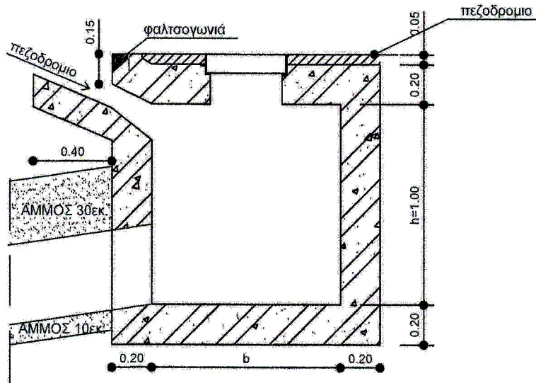
ΤΟΜΗ Α-Α ΣΤΟ ΠΕΖΟΔΡΟΜΙΟ
