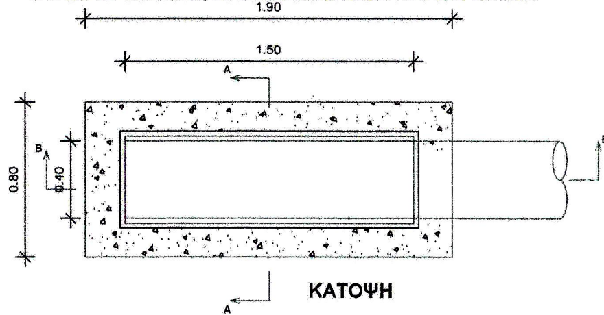
ΦΡΕΑΤΙΟ ΥΔΡΟΣΥΛΛΟΓΗΣ, ΤΟΠΟΘΕΤΟΥΜΕΝΟ ΚΑΘΕΤΑ ΣΤΟ ΟΡΙΟ ΤΗΣ ΟΔΟΥ
