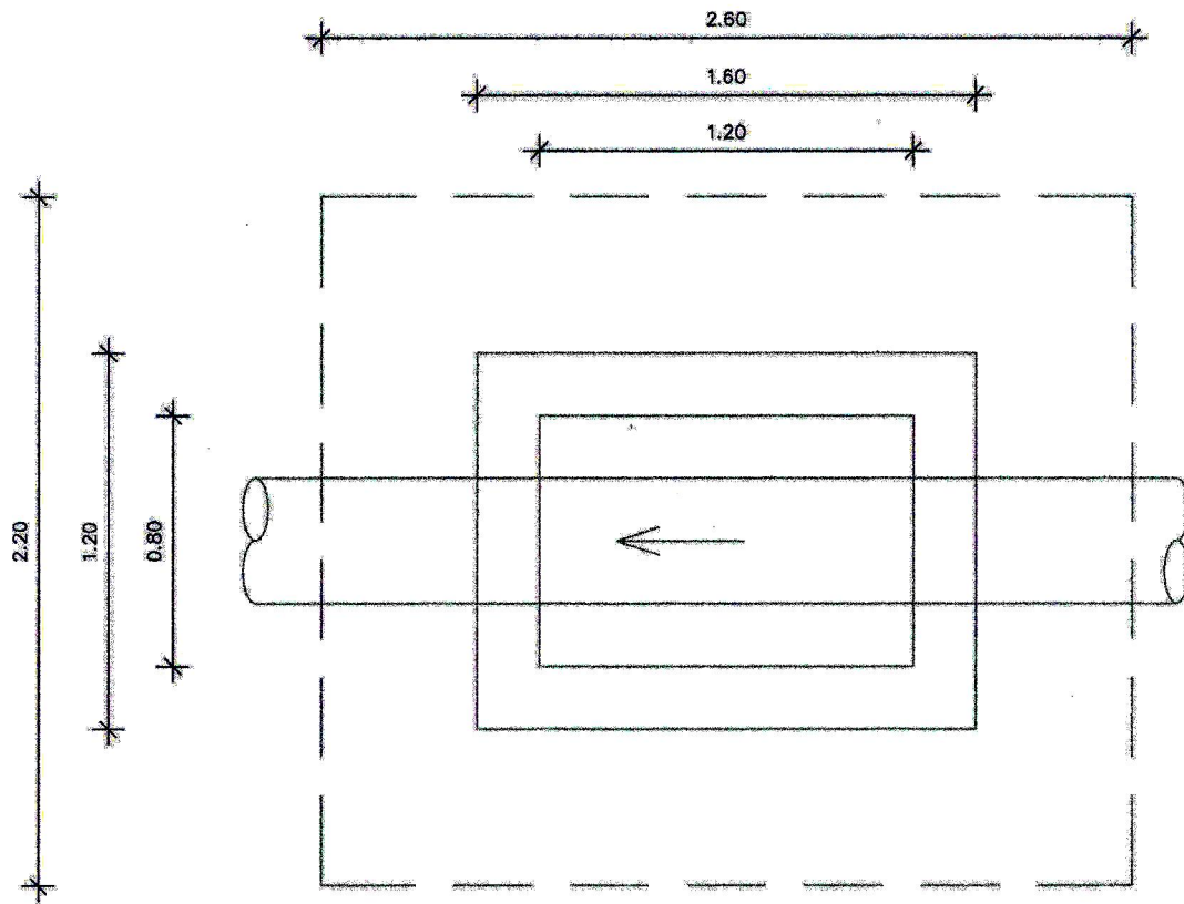
ΚΑΤΟΨΗ ΦΡΕΑΤΙΟΥ ΕΠΙΣΚΕΨΗΣ (ID<0.80)
