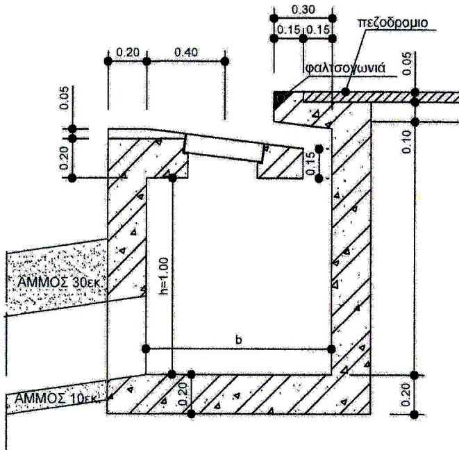
ΤΟΜΗ Α-Α ΣΤΟ ΟΔΟΣΤΡΩΜΑ
