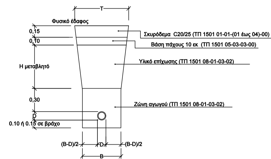
ΣΚΑΜΜΑ ΑΓΩΓΟΥ ΣΕ ΤΣΙΜΕΝΟΣΤΡΩΜΕΝΗ ΟΔΟ
