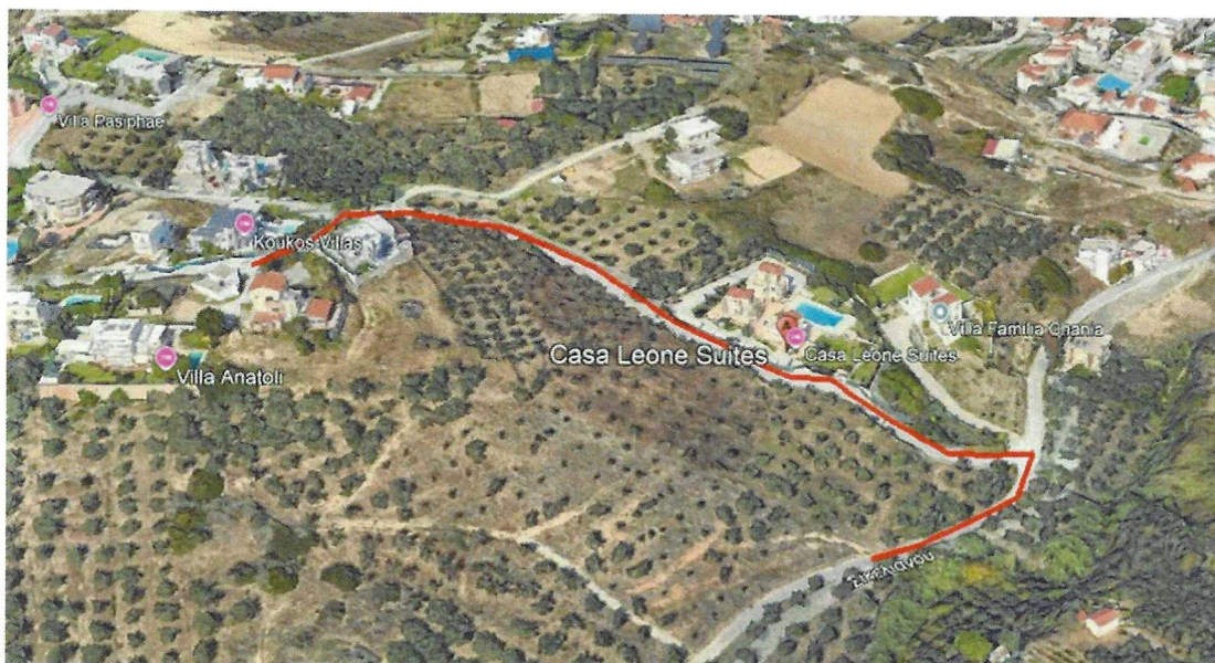
Κάτω Σταλός, αγωγός ονομ. διαμέτρου DN 110 mm 16 atm συνολικού μήκους 370 μ
